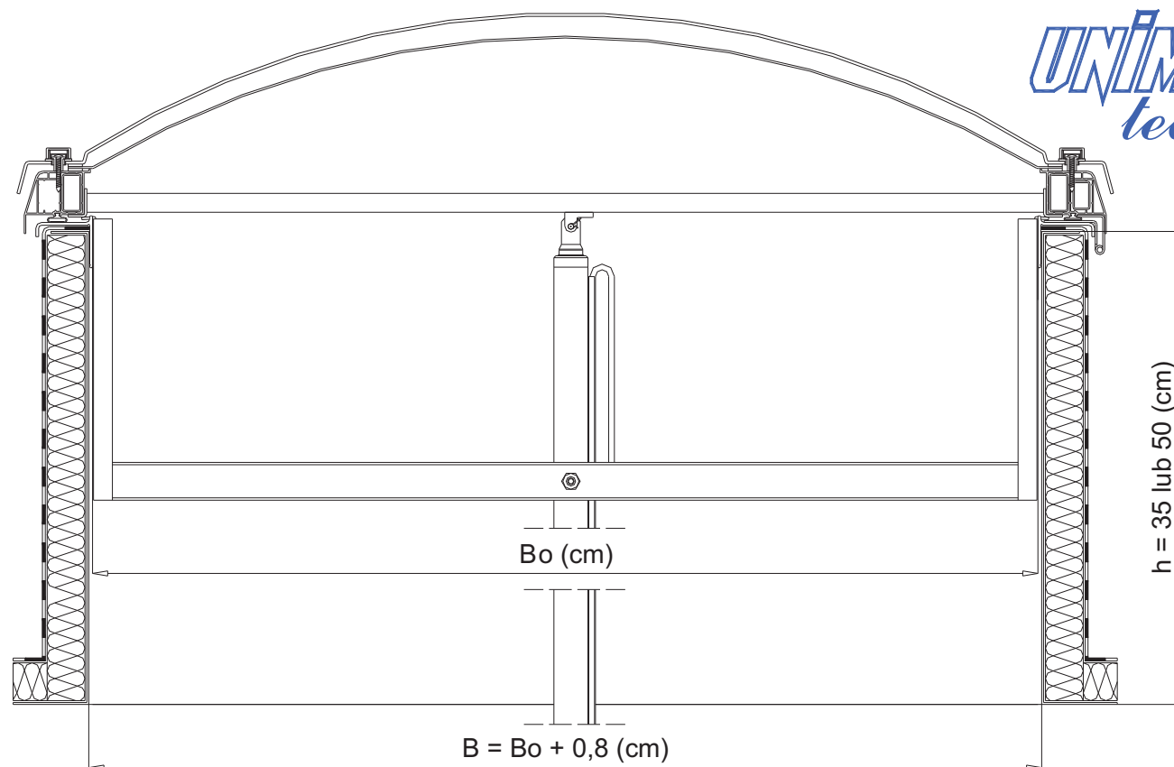
rys. UPI 01-11 – KLAPA DYMOWA NA PODSTAWIE PROSTEJ STEROWANIE ODDYMIANIEM I PRZEWIETRZANIEM – ELEKTRYCZNE 24 V DC
