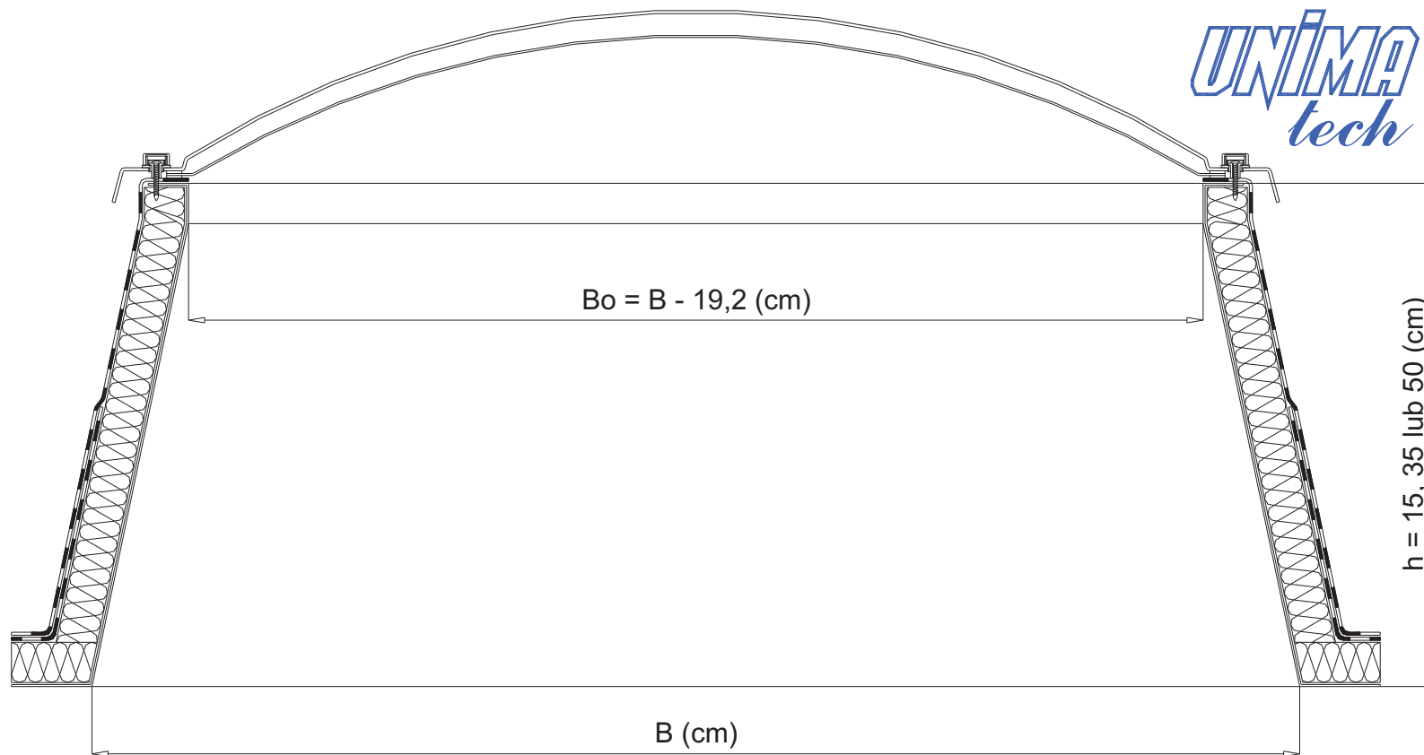
rys. UPI 02-01 – ŚWIETLIK STAŁY NA PODSTAWIE SKOŚNEJ
