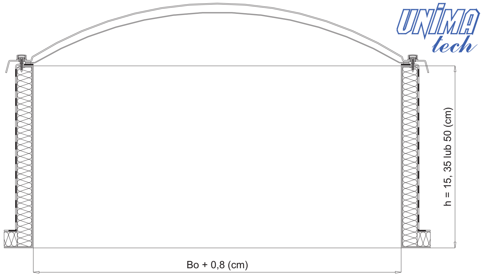
rys. UPI 02-02 – ŚWIETLIK STAŁY NA PODSTAWIE PROSTEJ
