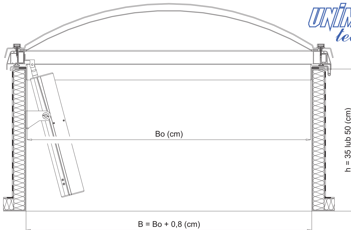
rys. UPI 02-04 – ŚWIETLIK OTWIERANY NA PODSTAWIE PROSTEJ STEROWANIE PRZEWIETRZANIEM – ELEKTRYCZNE 230 V AC
