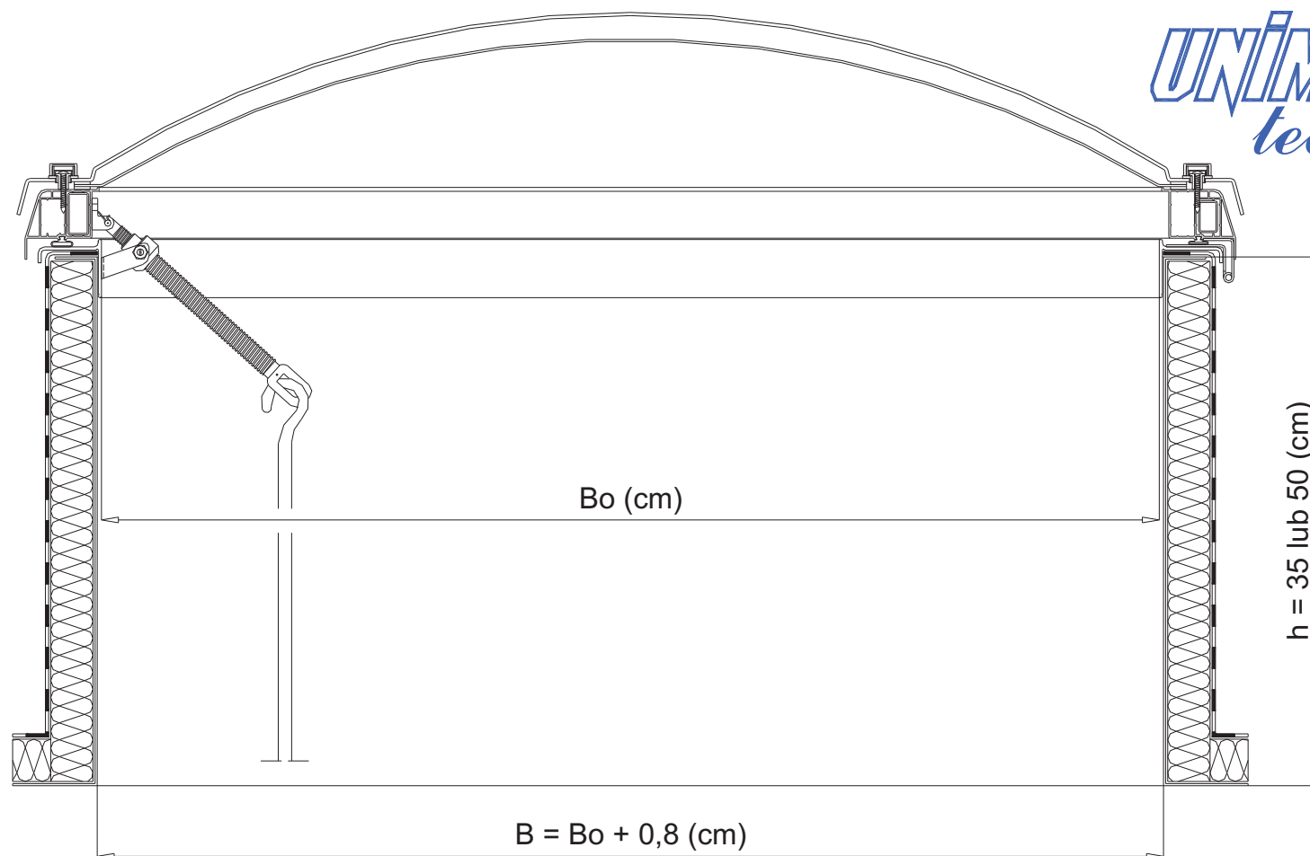
rys. UPI 02-06 – ŚWIETLIK OTWIERANY NA PODSTAWIE PROSTEJ STEROWANIE PRZEWIETRZANIEM – RĘCZNE
