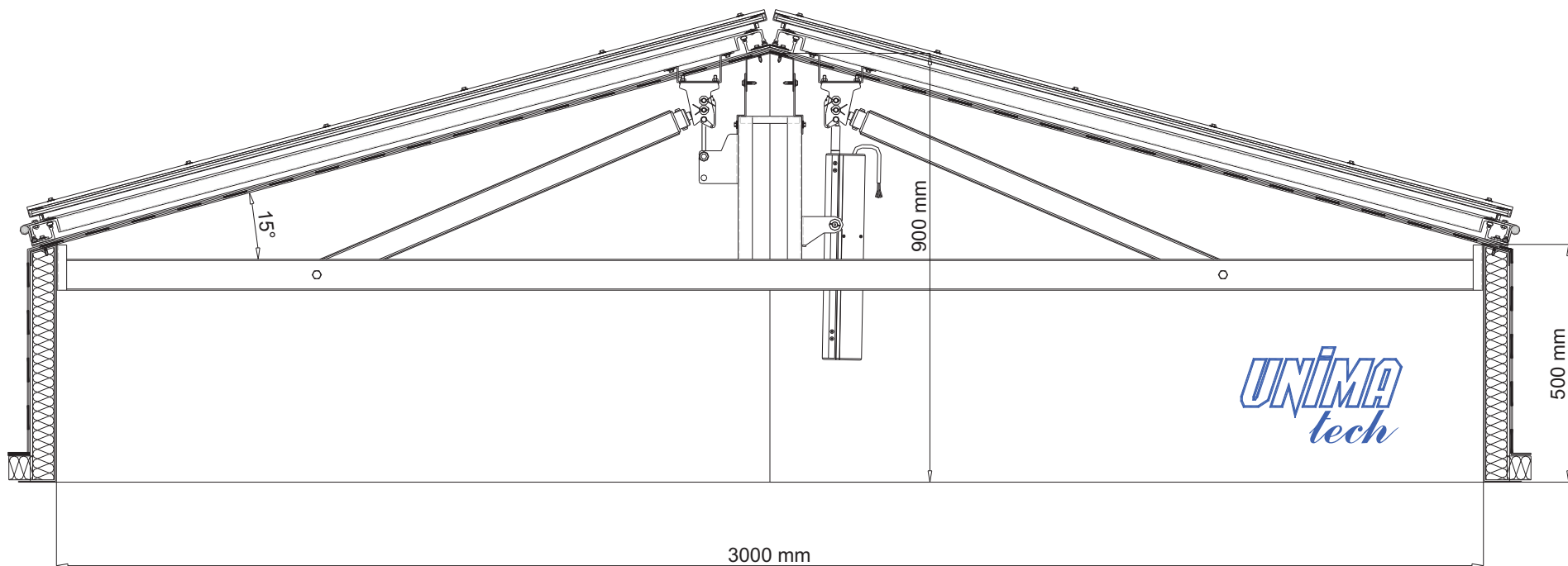
rys. UPI 03-03 – KLAPA DYMOWA 2,00x3,00 m ODDYMIANIE – PNEUMATYCZNE PRZEWIETRZANIE JEDNEGO SEGMENTU – ELEKTRYCZNE 230 V AC STAN ZAMKNIĘTY
