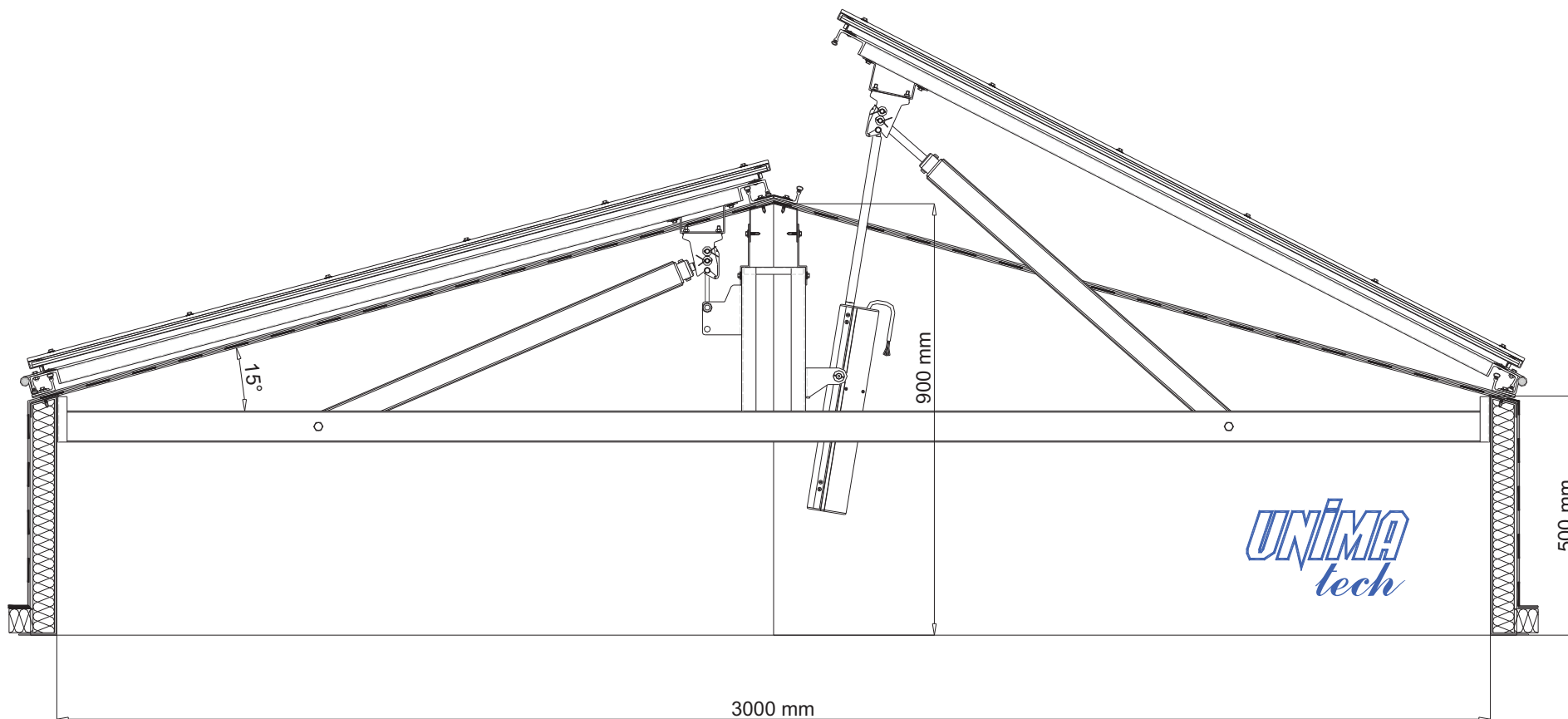
rys. UPI 03-05 – KLAPA DYMOWA 2,00x3,00 m ODDYMIANIE – PNEUMATYCZNE PRZEWIETRZANIE JEDNEGO SEGMENTU – ELEKTRYCZNE 230 V AC PRZEWIETRZANIE – STAN OTWARTY
