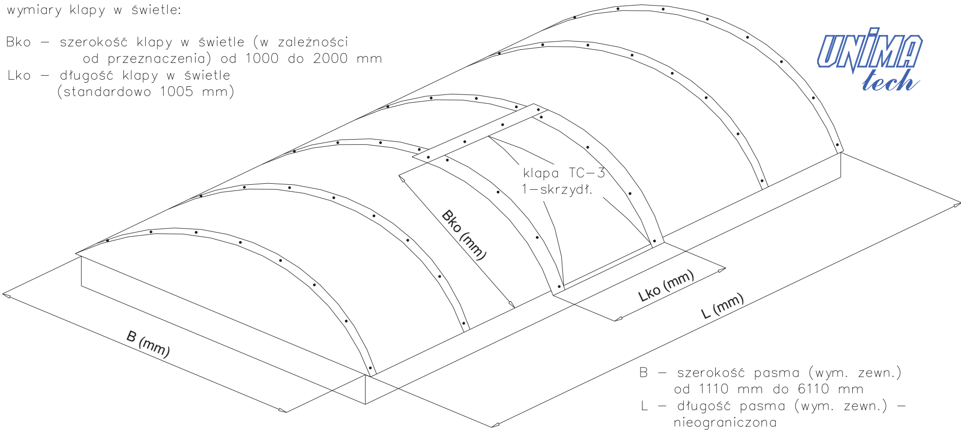
rys. UPI 04-02 – PASMO ŚWIETLNE ŁUKOWE Z KLAPĄ JEDNOSKRZYDŁOWĄ TC-3
