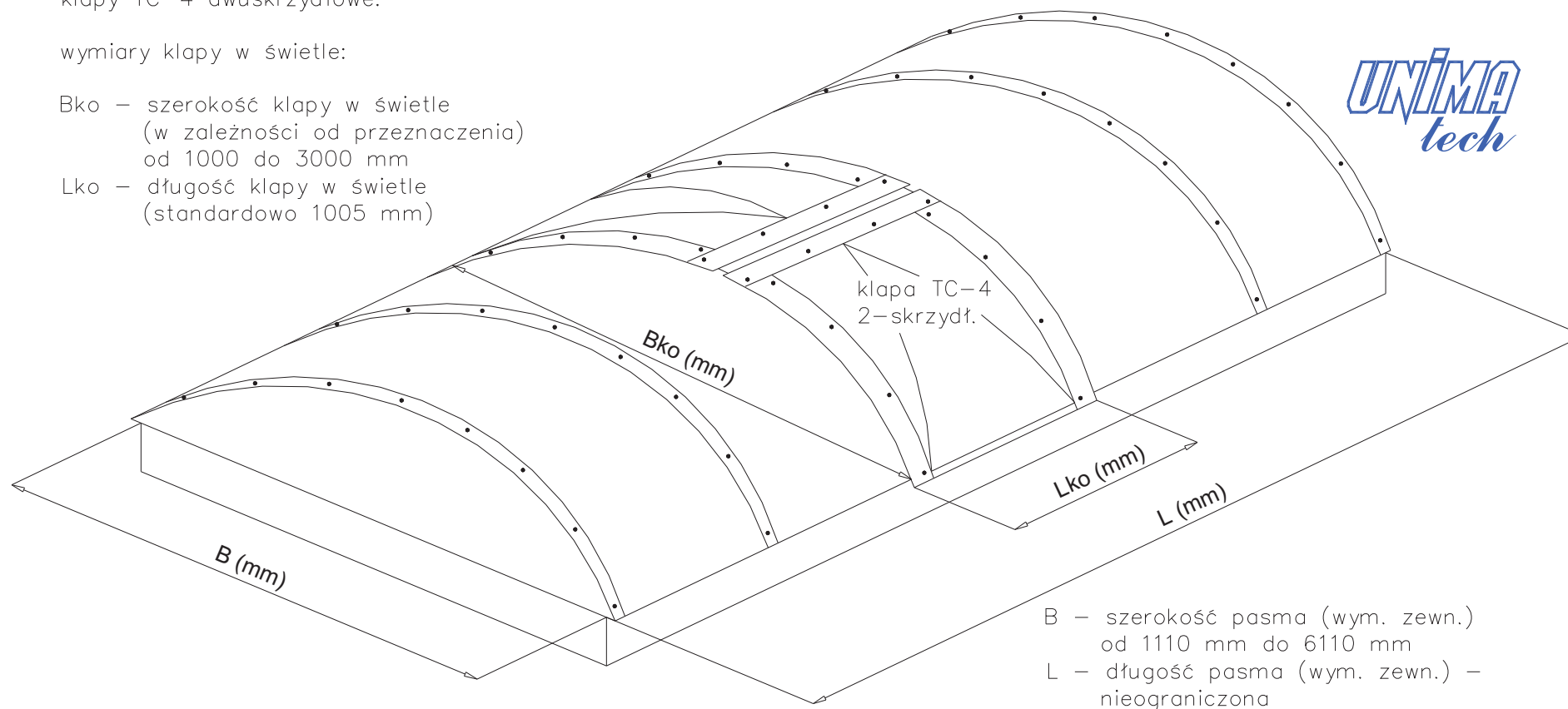
rys. UPI 04-03 – PASMO ŚWIETLNE ŁUKOWE Z KLAPĄ DWUSKRZYDŁOWĄ TC-4
