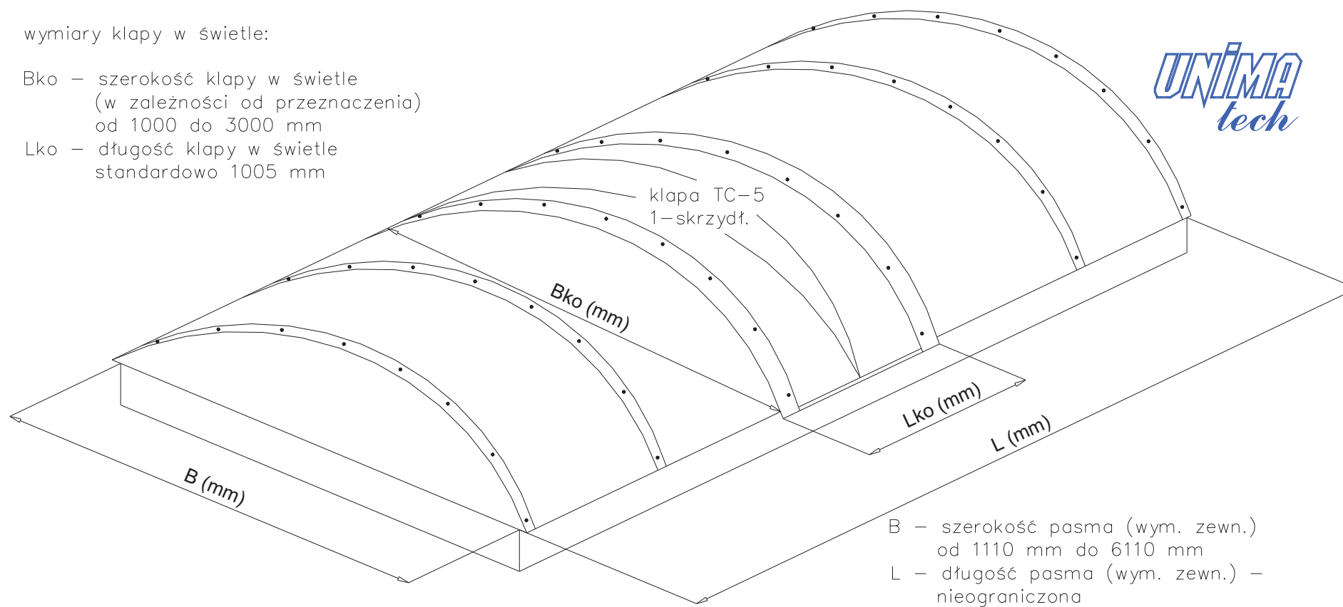
rys. UPI 04-04 – PASMO ŚWIETLNE ŁUKOWE Z KLAPĄ JEDNOSKRZYDŁOWĄ TC-5
