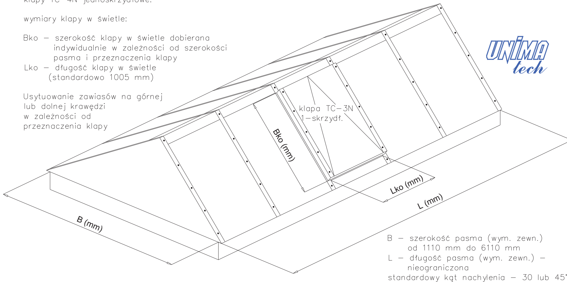
rys. UPI 04-10 – PASMO ŚWIETLNE TRÓJKĄTNE Z KLAPĄ JEDNOSKRZYDŁOWĄ TC-3N
