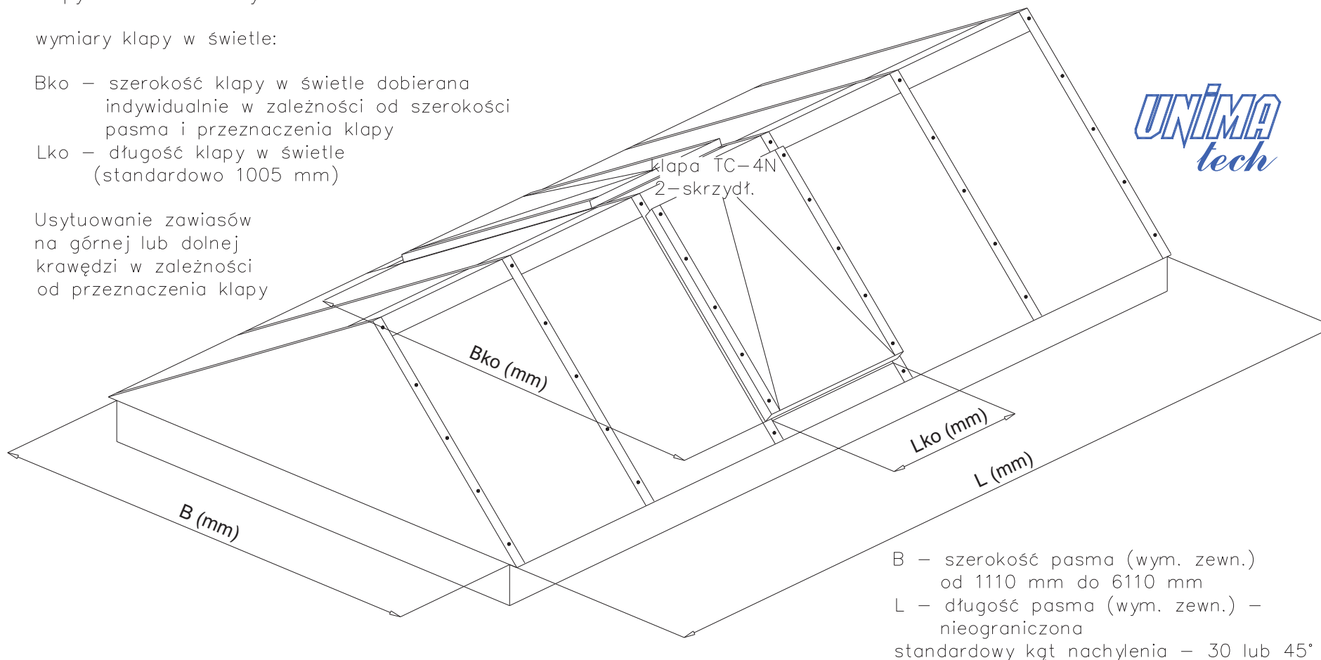
rys. UPI 04-11 – PASMO ŚWIETLNE TRÓJKĄTNE Z KLAPĄ DWUSKRZYDŁOWĄ TC-4N
