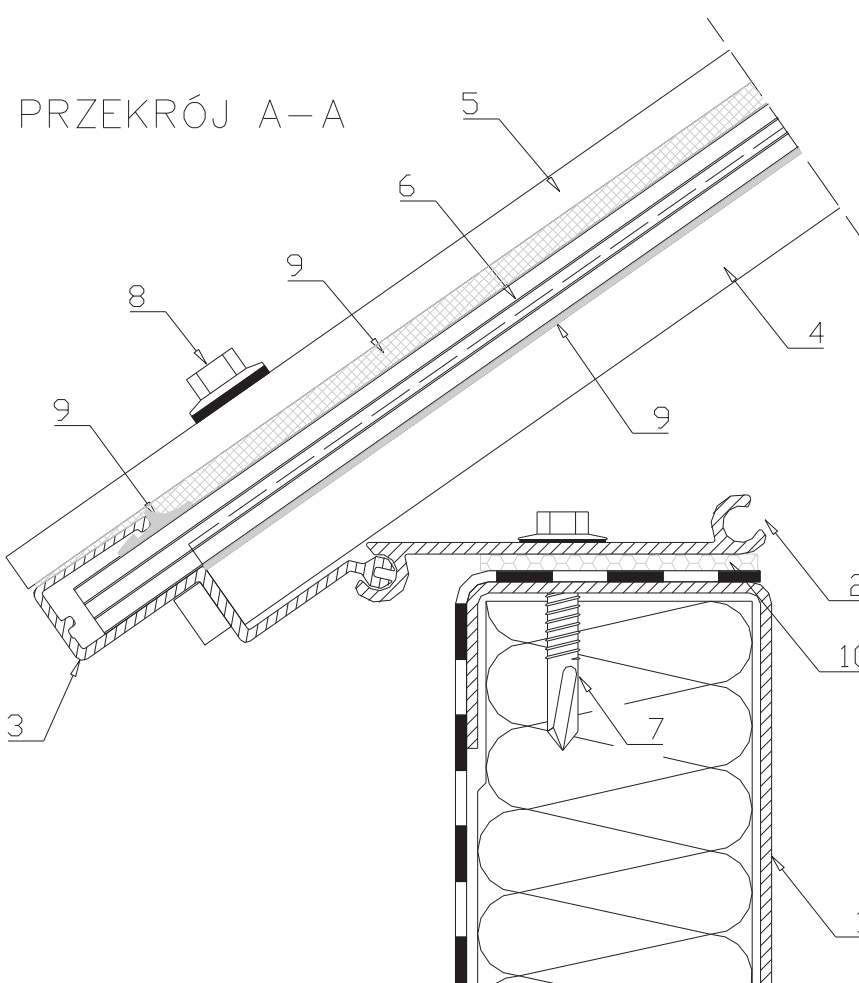
rys. UPI 09-02 – PRZEKRÓJ PRZEZ PROFIL ŁAPKOWY – PRZYKŁAD 1
