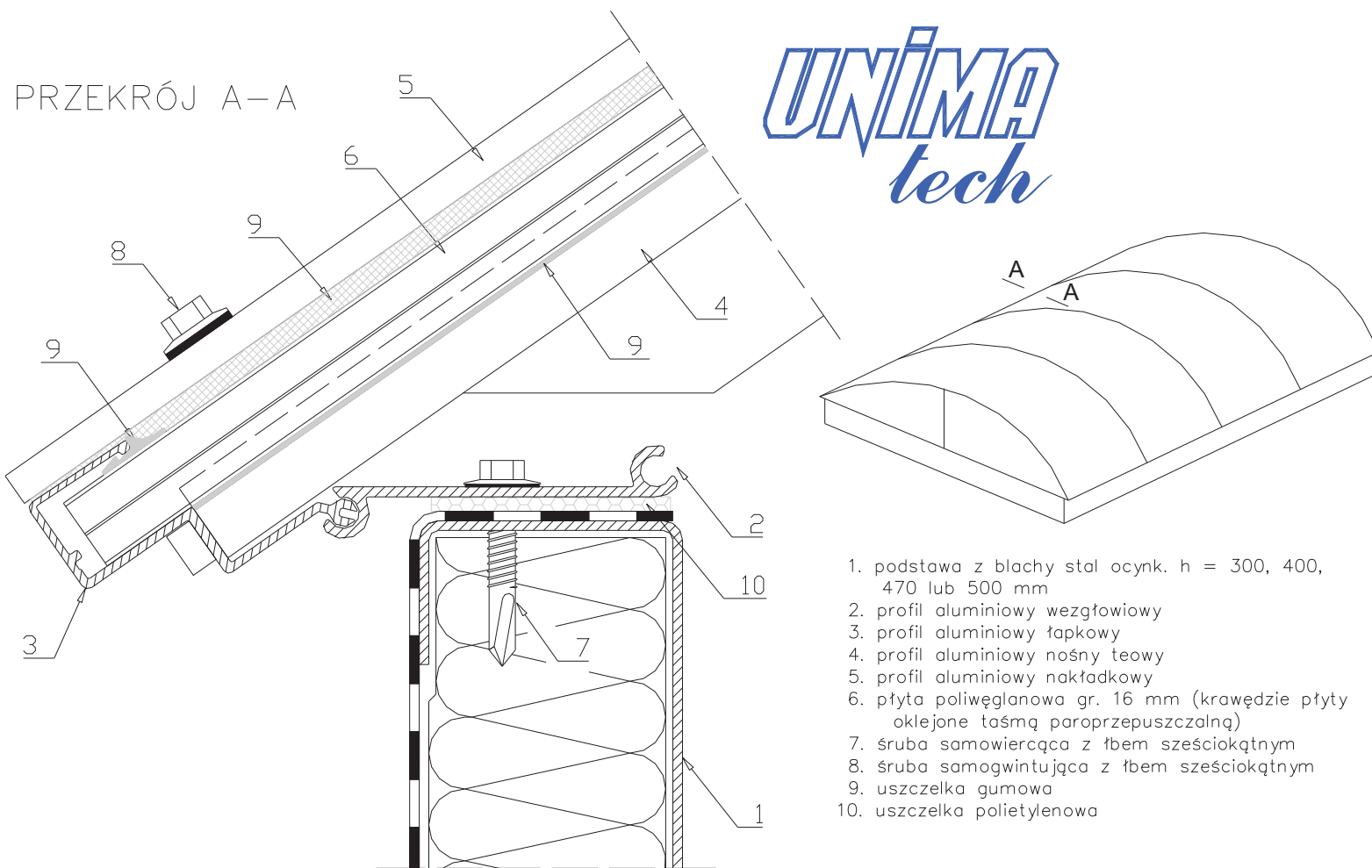
rys. UPI 09-03 – PRZEKRÓJ PRZEZ PROFIL ŁAPKOWY – PRZYKŁAD 2
