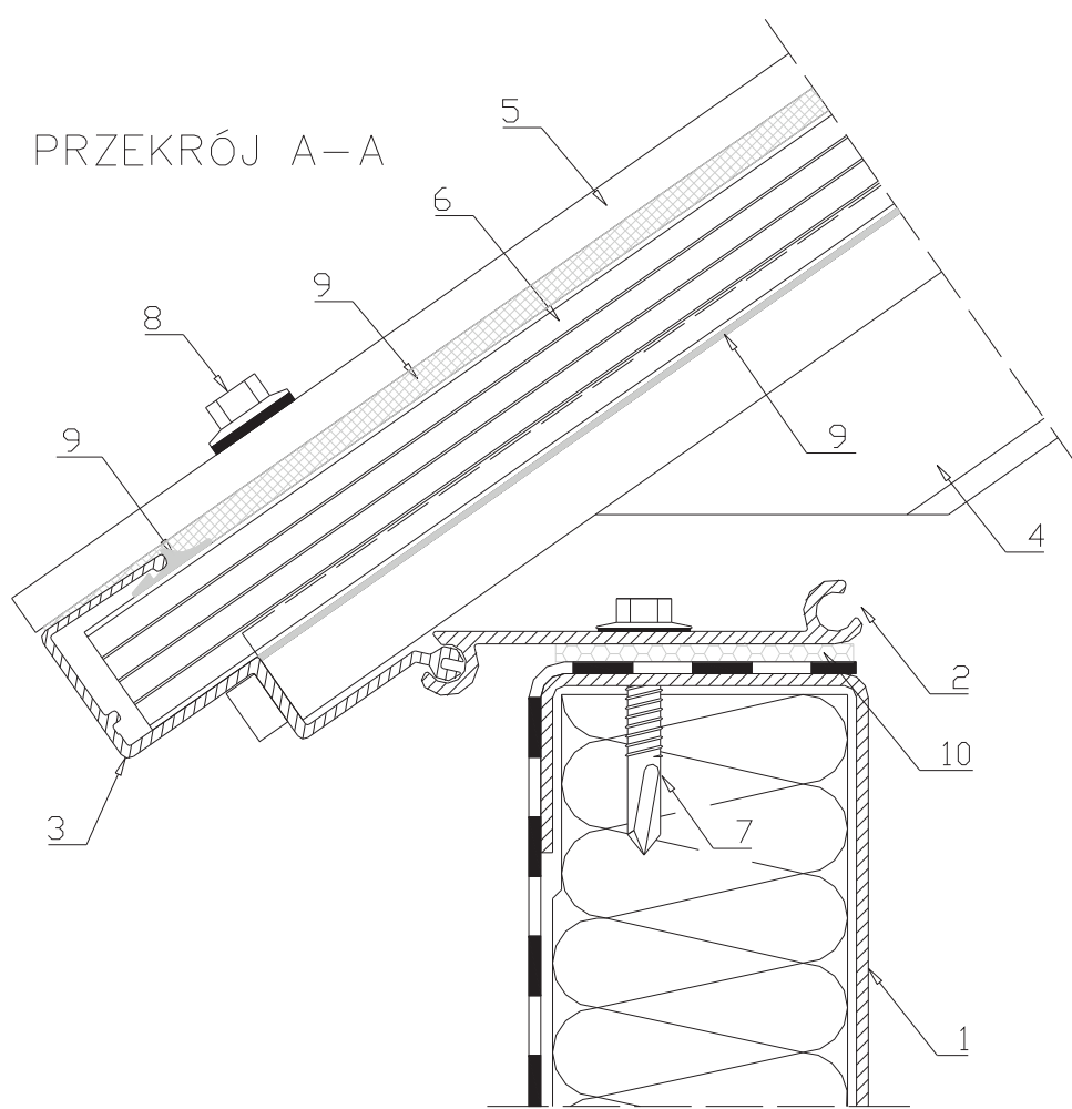
rys. UPI 09-04 – PRZEKRÓJ PRZEZ PROFIL ŁAPKOWY – PRZYKŁAD 3
