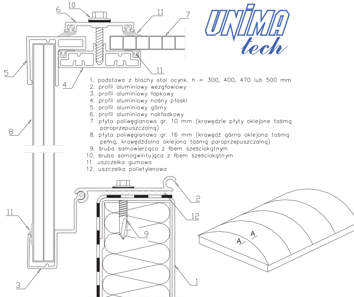
rys. UPI 11-02 – ZAKOŃCZENIE PASMA "PEŁNY KONIEC" – PRZYKŁAD 1
