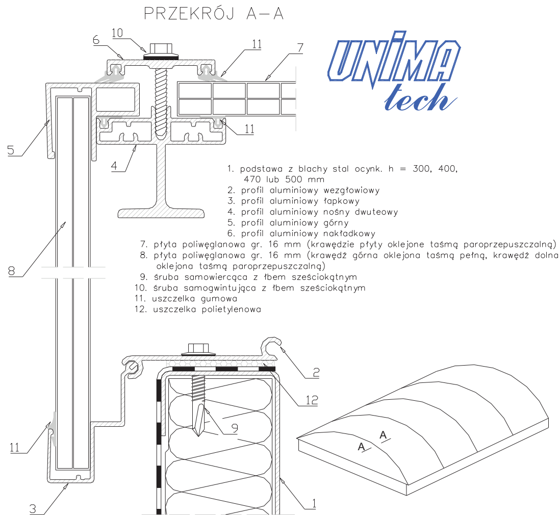
rys. UPI 11-04 – ZAKOŃCZENIE PASMA "PEŁNY KONIEC" – PRZYKŁAD 3
