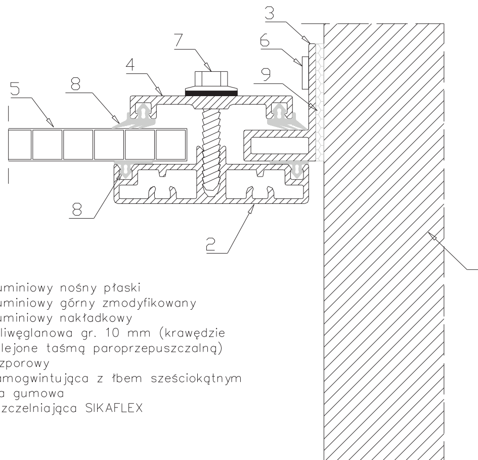
PRZEKRÓJ A-A
