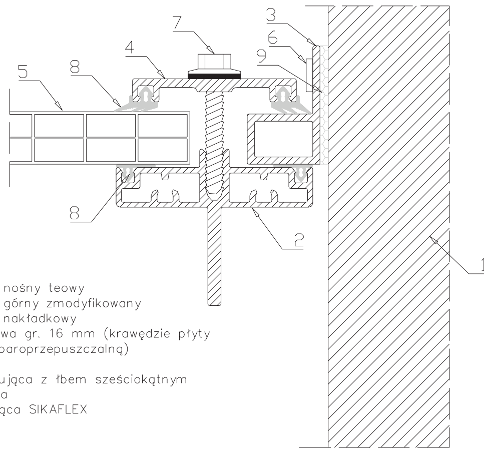
rys. UP 12-03 – ZAKOŃCZENIE PASMA "STYK Z MUREM" – PRZYKŁAD 2
