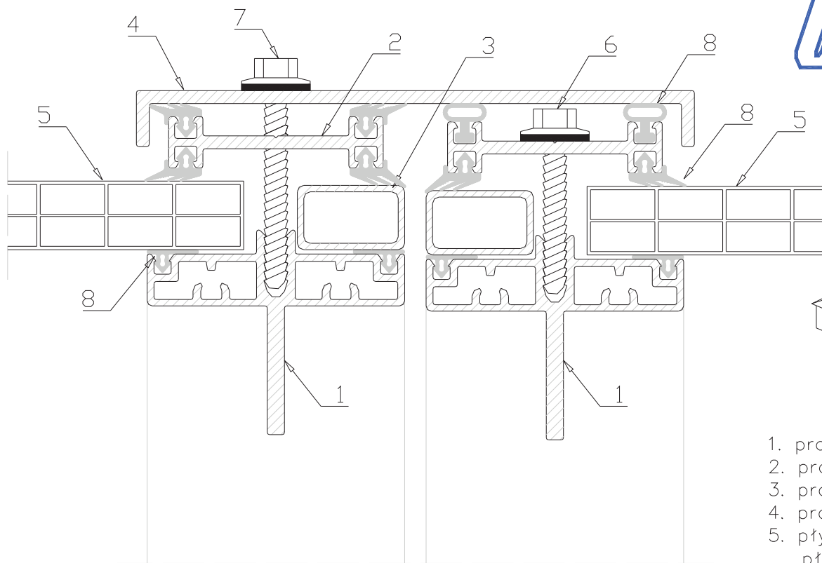
rys. UPI 14-02 – KLAPA TC – PRZEKRÓJ PODŁUŻNY
