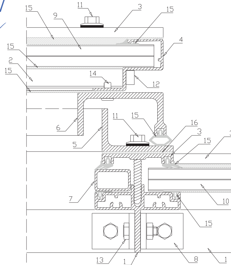
rys. UP 15-04 - KLAPA KD - STRONA PRZECIWSZAWIASOWA
